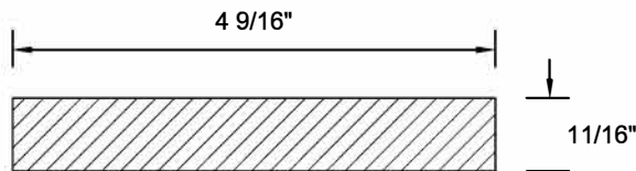
#2335 DOOR JAMB
